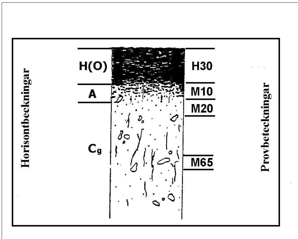
Fig. 11.7.24.4 Exempel på horisont- och provbeteckningar – Gleysol.
