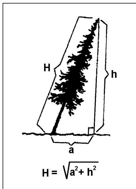
Fig. B1.2 Om trädet lutar starkt ( > 10^\circ ) mäts avståndet från marken till toppen ( h ). Därefter lodar man in den punkt som ligger rakt under trädets topp och mäter avståndet från denna till trädet ( a ). Trädets rätta höjd ( H ) beräknas som hypotenusan i en rätvinklig triangel, där kateterna ( a och h ) är kända.
